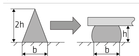
Abbildung 1: Empfohlener Klebstoffauftrag
