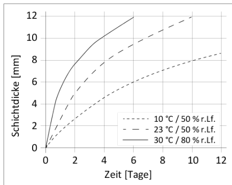
Diagramm 1: Durchhärtgeschwindigkeit Sikaflex®-268
