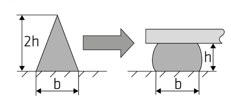
Abbildung 1: Empfohlener Klebstoffauftrag
