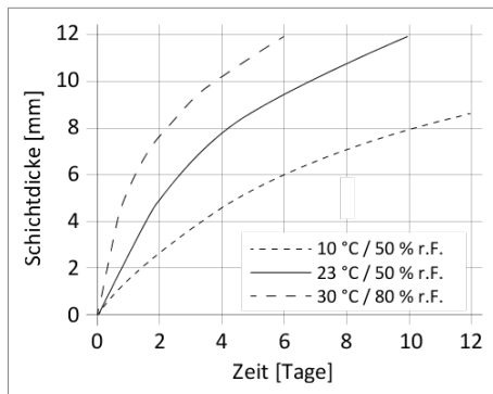
Diagramm 1: Durchhärtengeschwindigkeit Sikaflex®-252
