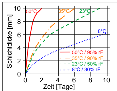
Diagramm 1: Durchhärtegeschwindigkeit von 1 Komponenten-Sikasil®
