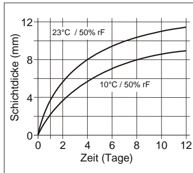
Diagramm 1: Durchhärtungsgeschwindigkeit für Sikaflex®290i DC
